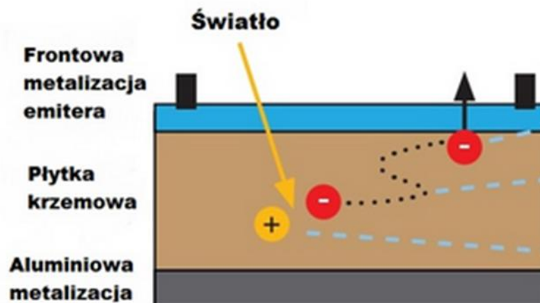
Rysunek nr 2. Budowa i zasada działania ogniwa
